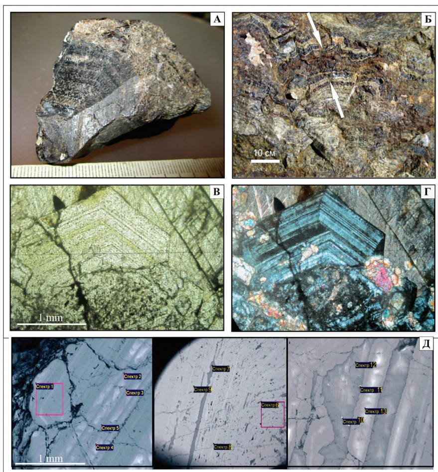
Рис. 2. Зональность гранатов месторождения Алексеевское: а, б – макрозональность (стрелками показано направление роста); в-г – микрозональность (шлиф, без анализатора и с анализатором); д – изображение в BSE.
