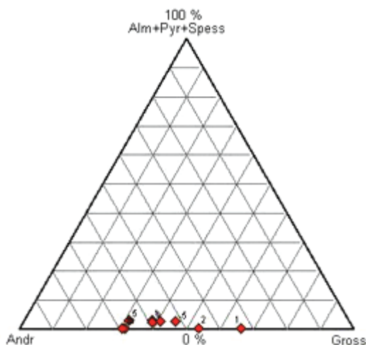
Рис. 3. Составы зональных гранатов месторождений Северной Хакасии.
