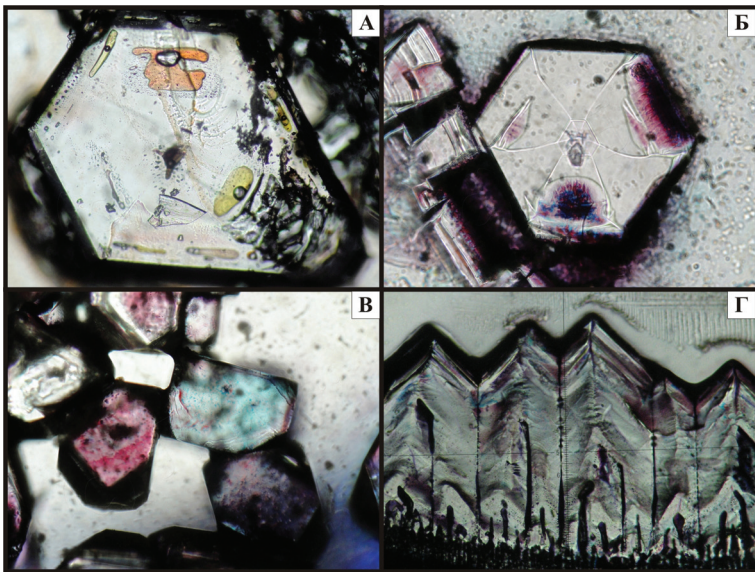
Рис. 1. Зональность в кристаллах алюмокалиевых квасцов: а – кристалл с жидкими включениями (красного и жёлтого цвета); б, в – кристаллы, избирательно включившие пищевые красители; г – геометрический отбор кристаллов алюмокалиевых квасцов (величиной 0,1 – 1 мм).
